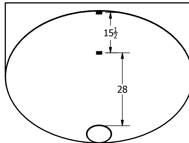
SECTION A-A SCALE 1:22
